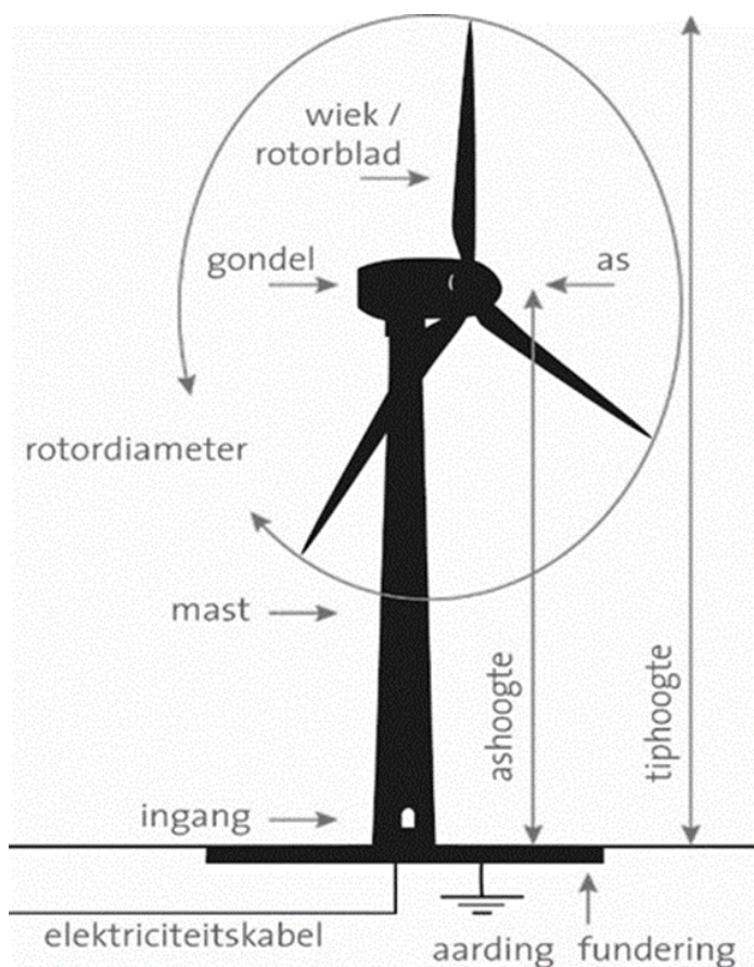
Figuur 4.2 Turbine-aanduidingen
