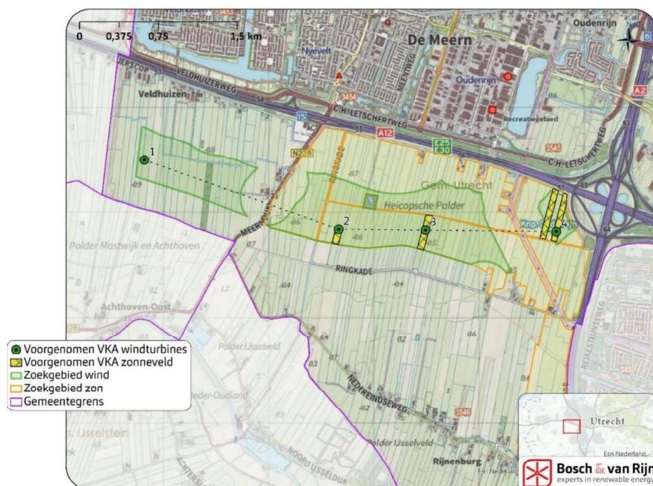
Figuur 1: plattegrond met posities van de vier windturbines
